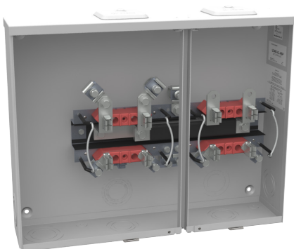
U3492-XL-HSP
