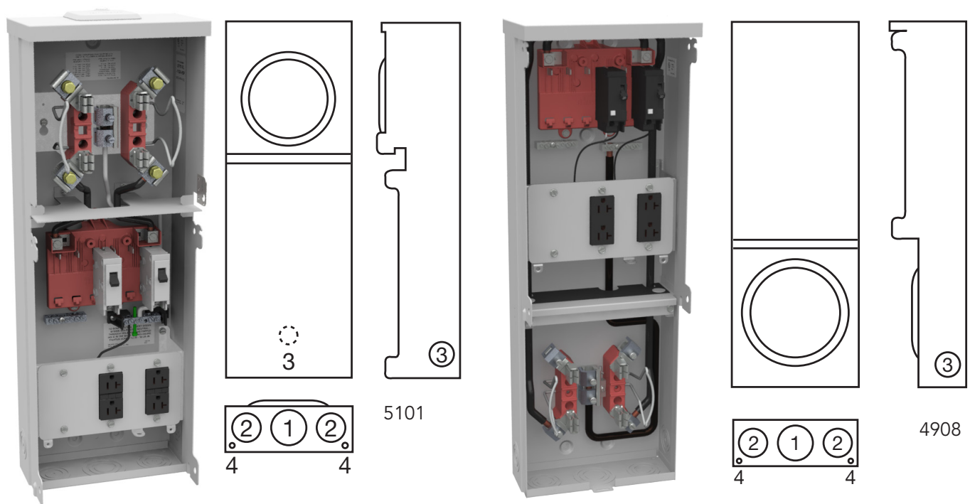
U5101-XL-100MB-11GR-HSP
