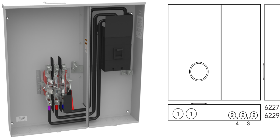
U6229-X-400-K7L
